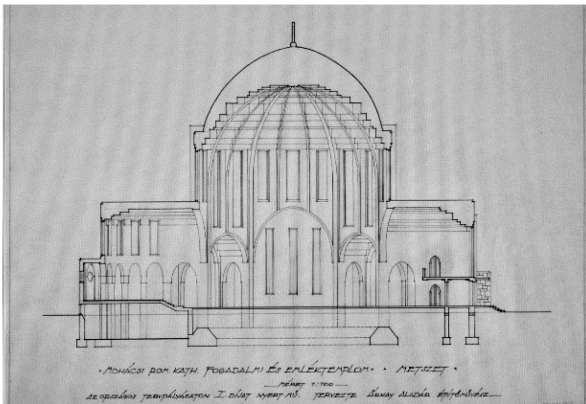
25. kép Metszet 29
