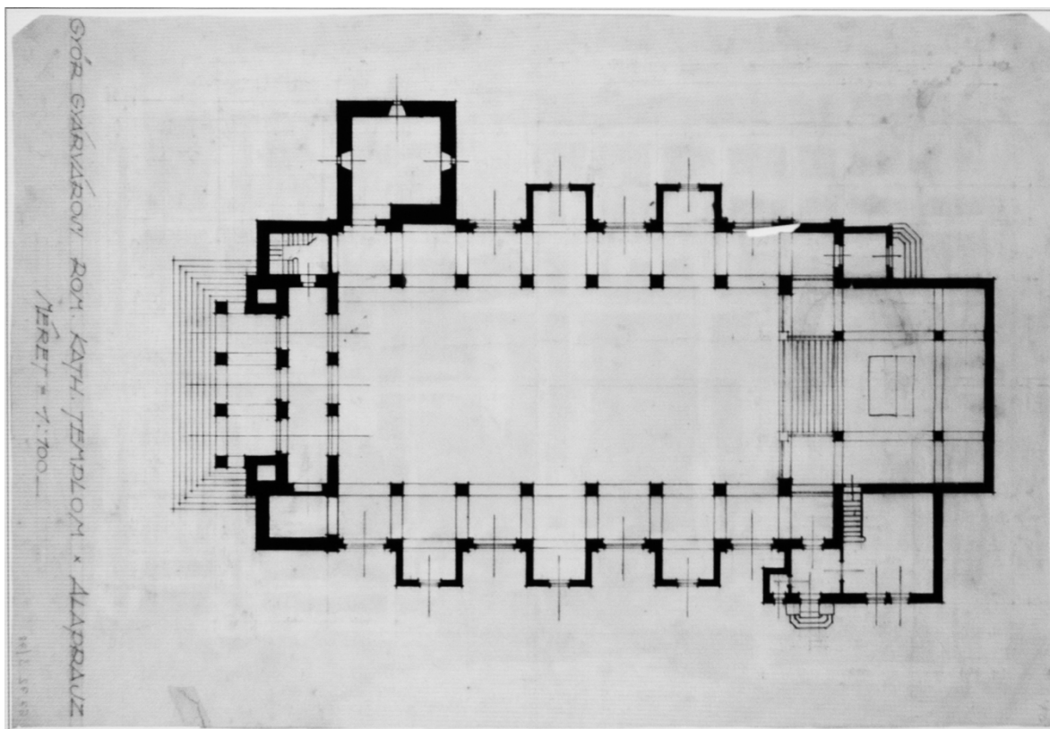
10. kép Alaprajz 12
