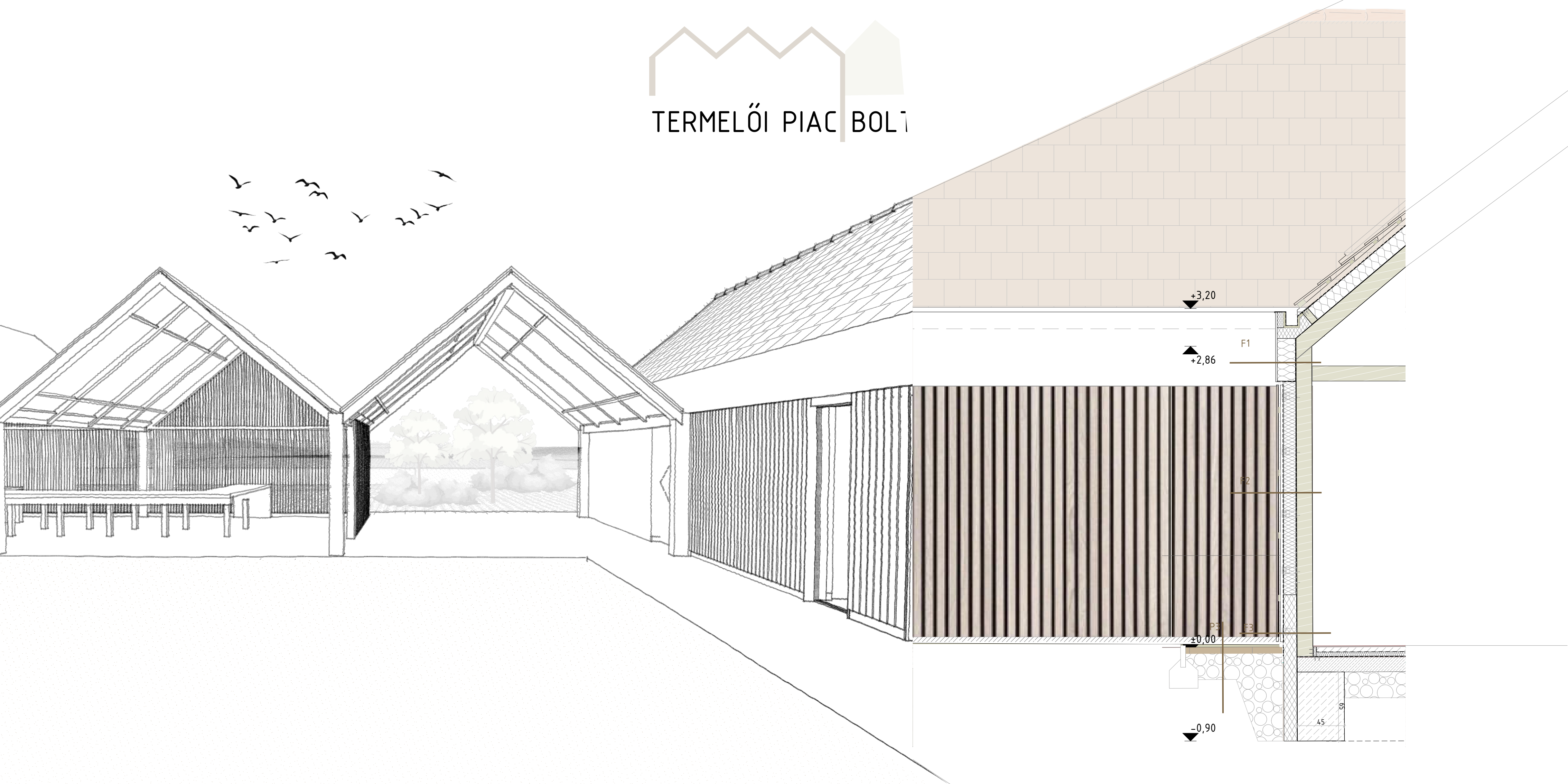
FALMETSZET 1:25
