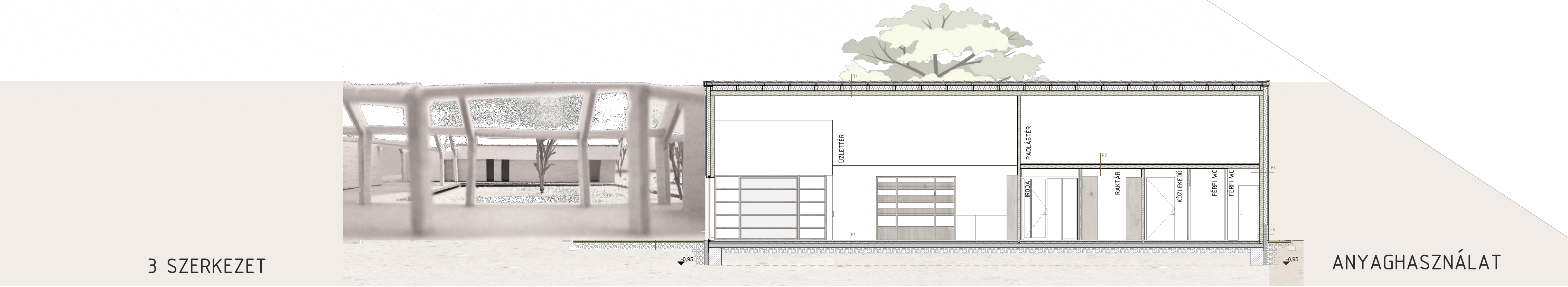
HOSSZMETSZET 1:100
