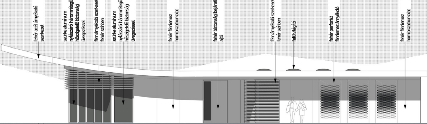
DÉLNYUGATI HOMLOKZATI 1:100
